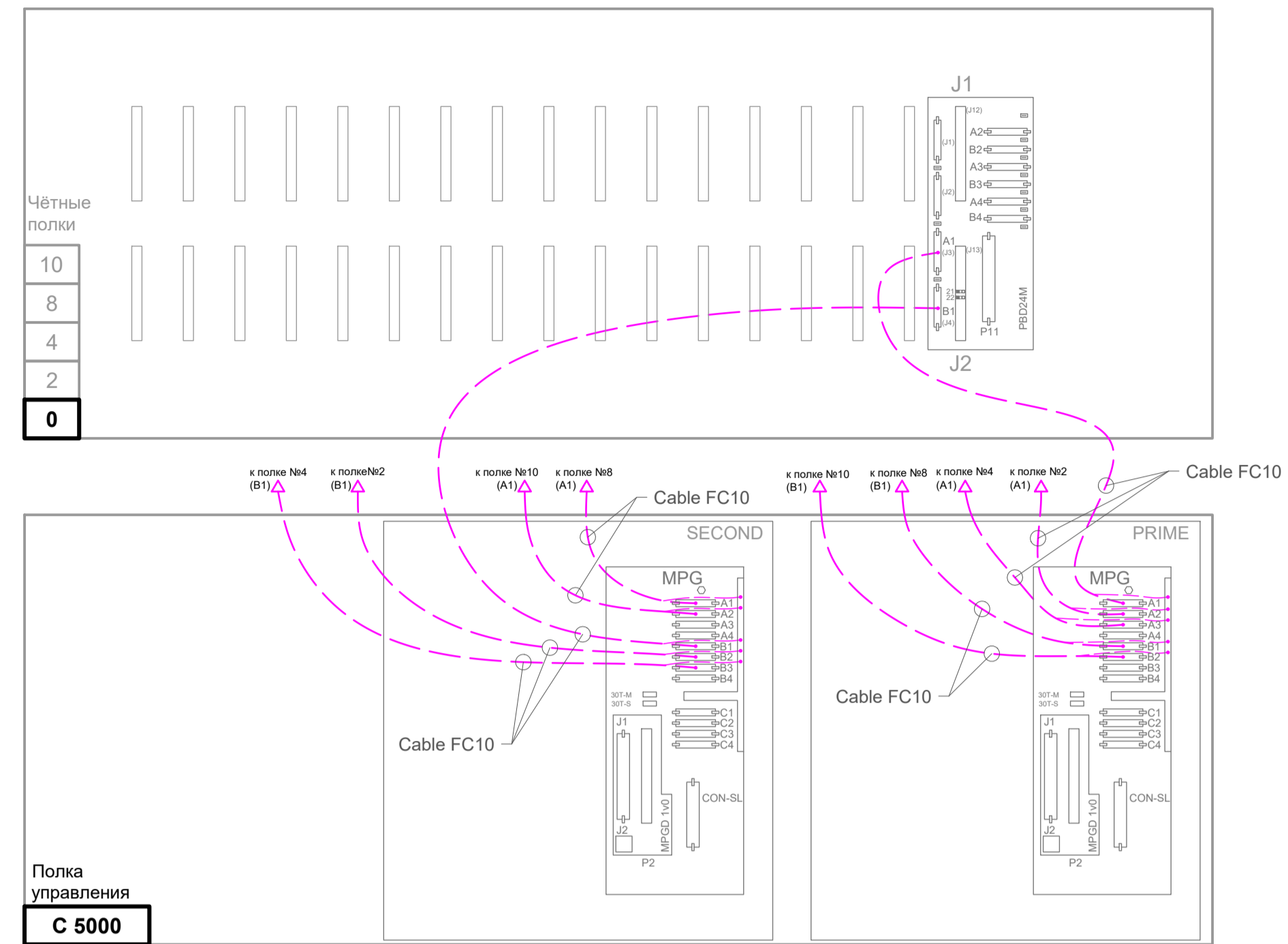
Схема подключения кабелей системы PCM&HDLC.
