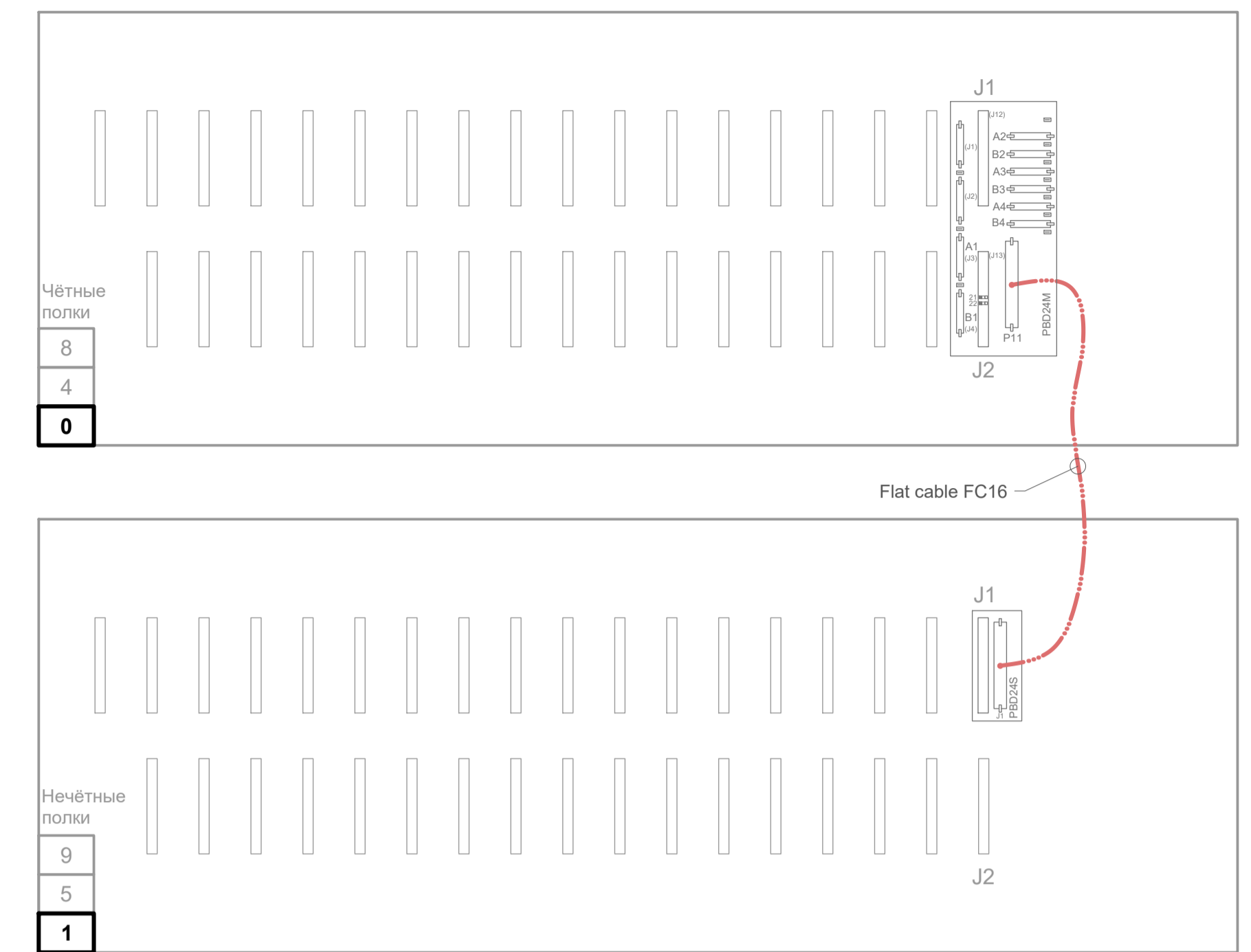
Схема подключения нечётных полок к чётным.
