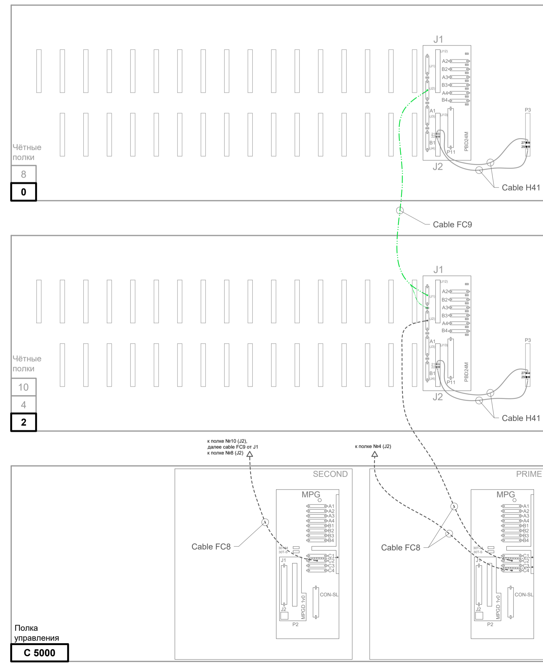
Схема подключения кабелей системы Clock&Sync_Signal (FC9) и Alarm (H41).
