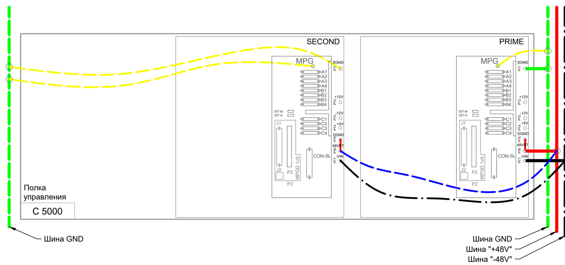
Схема подключения электропитания и заземления.
