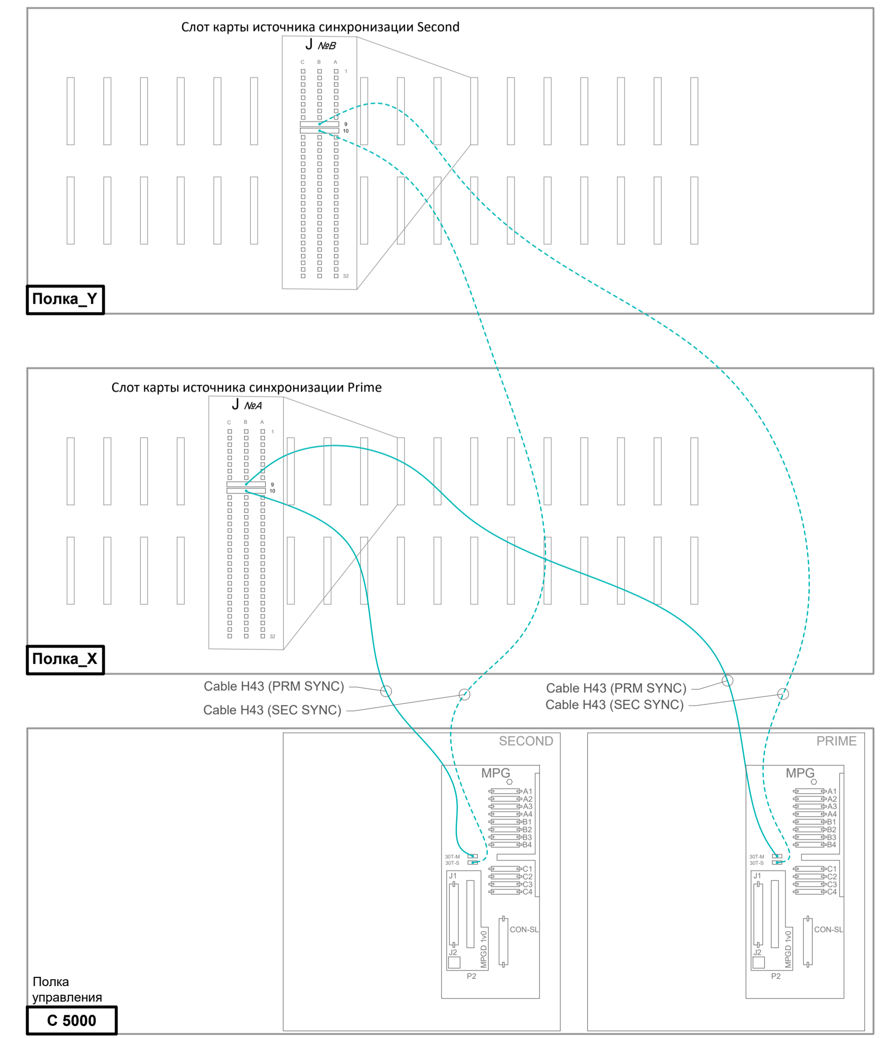
Схема подключения кабелей синхронизации.
