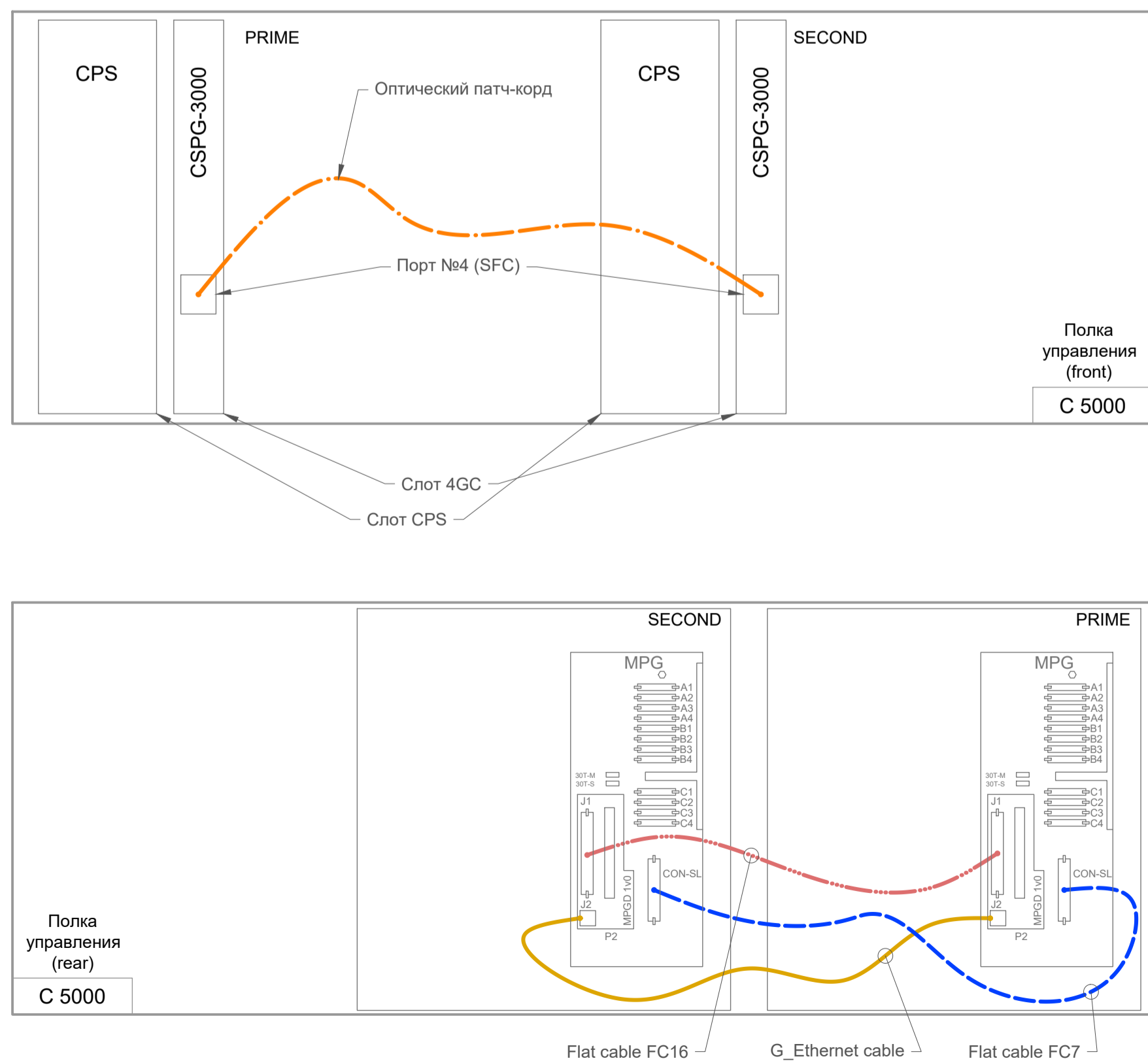
Контроль соединений кабелей системы "Суперлинк+".
